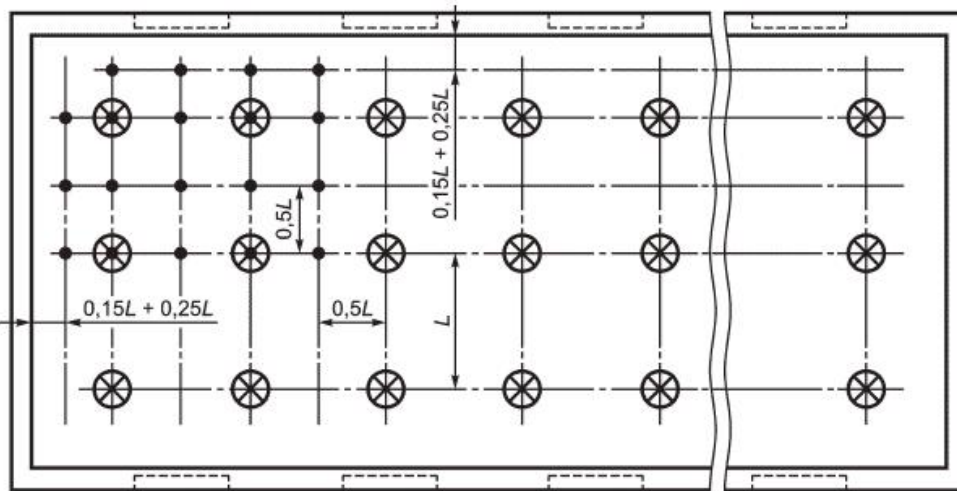
Рисунок А.1 - Расположение контрольных точек при измерении минимальной освещенности помещения от светильников, принимаемых за точечные излучатели
