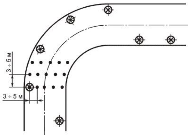
Рисунок А.7 - Расположение контрольных точек при измерении средней освещенности улиц в местах закругления
