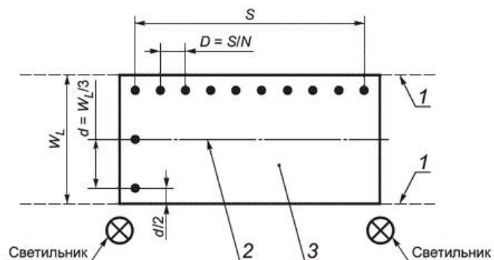
Рисунок А.5 - Расположение контрольных точек на участке при измерении средней освещенности улиц
