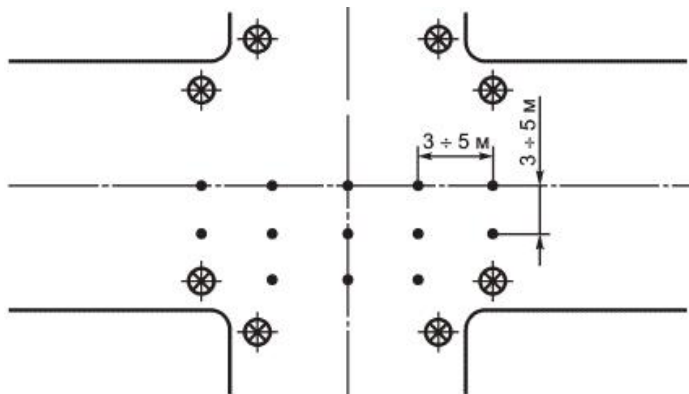
Рисунок А.6 - Расположение контрольных точек при измерении средней освещенности улиц на перекрестке
