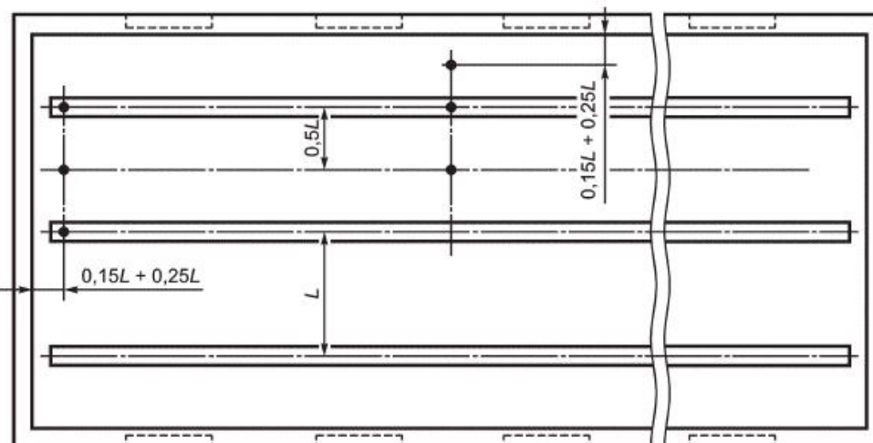
Рисунок А.2 - Расположение контрольных точек при измерении минимальной освещенности помещения от светильников, принимаемых за линейные излучатели
